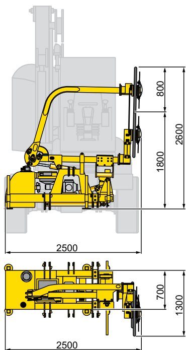
Ingombri in modalità trasferimento su strada Dimensions in transfer position
