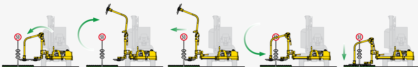
Ingombri in modalità trasferimento su strada Dimensions in transfer position
