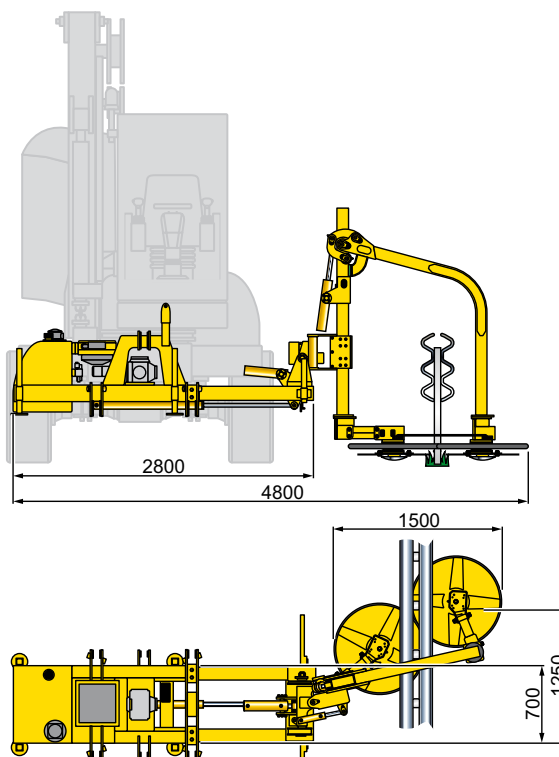
Ingombri in modalità lavoro Dimensions in working position
